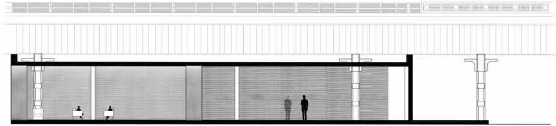
SECTION A SCALE: \frac{3}{16}'' = 1'-0''
