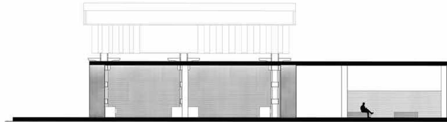
SECTION C SCALE: \frac{3}{16}'' = 1'-0''
